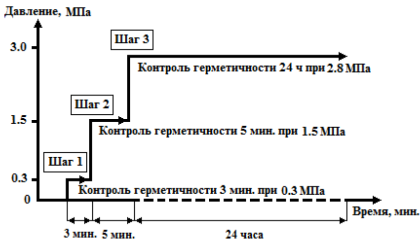
Рисунок 1 - Проверка герметичности азотом хладагентов R 22, R 407C
